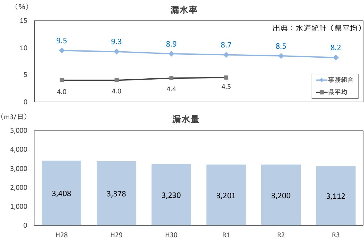
図 3-12 漏水状況
