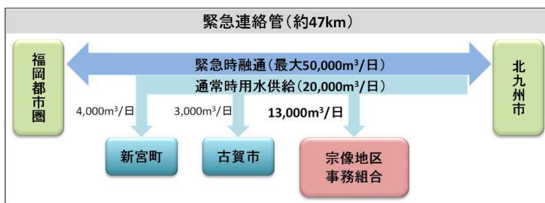
図 3-2 北部福岡緊急連絡管の水の流れ
