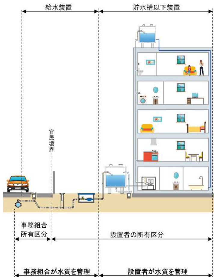
図 3-11 小規模貯水槽水道のしくみ
